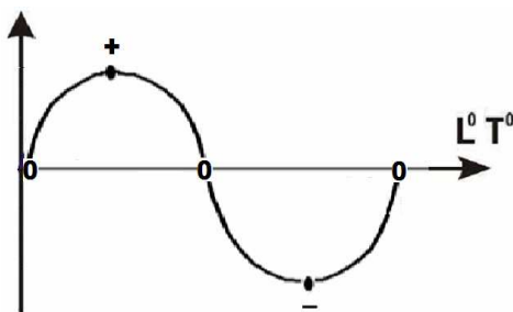
Рис. 3. Синусоидальная модель любого изменения
