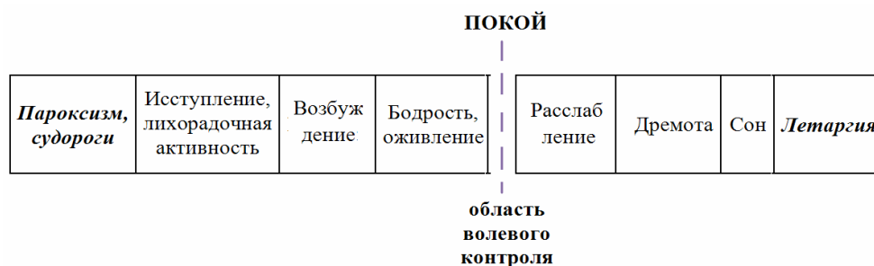
Рис. 1. Спектр переходов состояний психики
