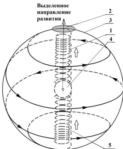
Рис. 9.3 – К рассмотрению процесса самоорганизации
