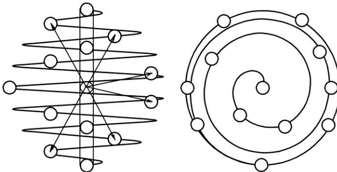
Рис. 7.33 – Схематическое изображение частицы согласно рассматриваемого процесса развития
