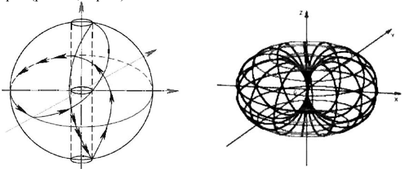
Рис. 6.3 – Сфера, проколота изолированным направлением, становится эквивалентом точки в классической геометрии (слева), а в трёхмерной интерпретации представлена тором (справа)
