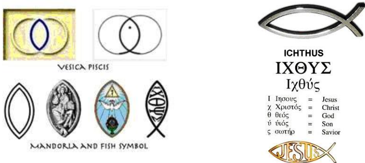
Рис. 8.8 – Связь символов Vesica piscis и Ιχθύς
