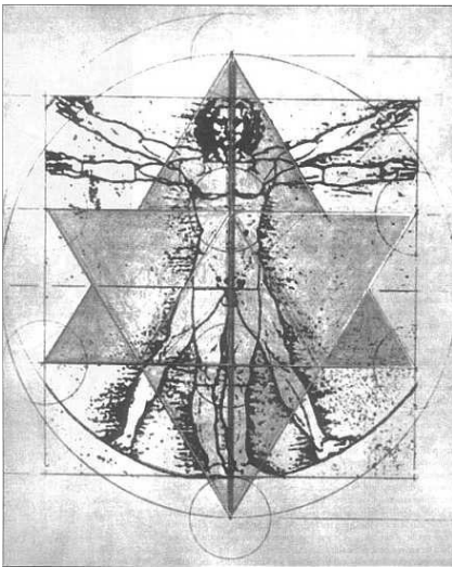
Рис. 6.20 – Рисунок Леонардо да Винчи с нанесенным на него звездным тетраэдром
