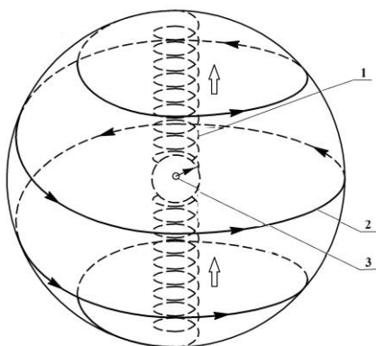
Рис. 9.1 – Схематическое изображение полного процесса одного уровня
