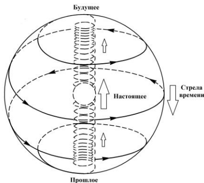
Рис. 6.7 – Направления развития внутренней и наружной спиралей
