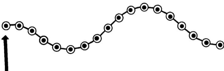
Рис. 7.12 – Колебания гибкой нити в свободном пространстве
