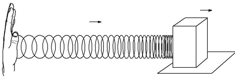
Рис. 9.4 – Схематическое объяснение эффекта телекинеза с помощью рассматриваемого процесса
