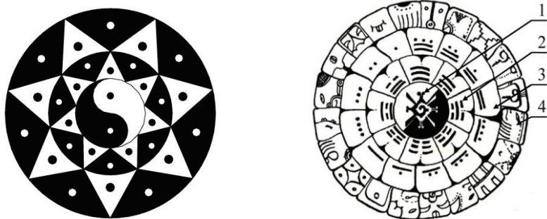
Рис. 6.19 – Геометрическая интерпретация кватернеров
