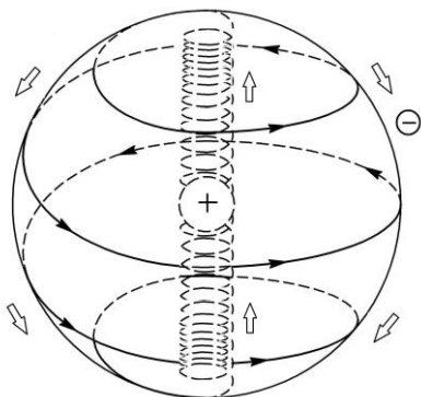
Рис. 7.7 – Элементарное вихревое поляризованное образование
