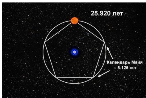
Рис. 8.37 – Определение продолжительности цикла Календаря Майя
