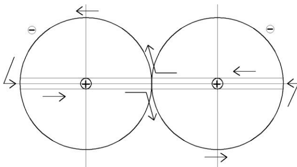
Рис. 7.25 – Схематическое изображение объединения обеих образований в единое целое вихревыми «восьмёрками»
