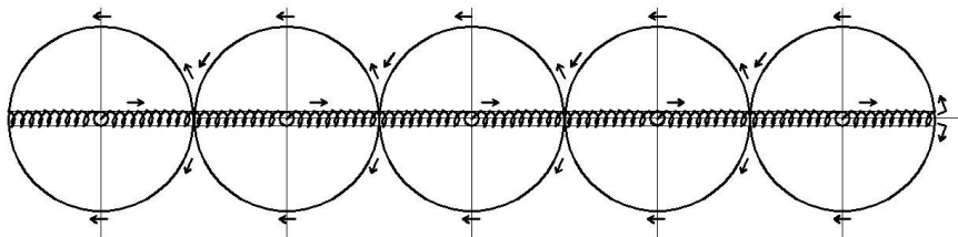
Рис. 7.8 – Схематическое изображение движения вихрей по поляризованной цепочке
