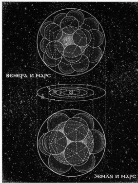
Рис. 8.35 – Геометрические взаимосвязи между орбитами Венеры и Марса, а также Земли и Марса
