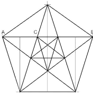
Рис. 8.7 – Пентаграмма – эмблема пифагорийцев
