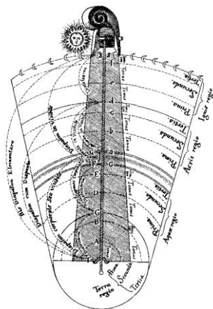
Рис. 6.11 – Монохорд с одной струной, прикрепленный верхним концом к Великому духу, а нижним – к абсолютной материи
