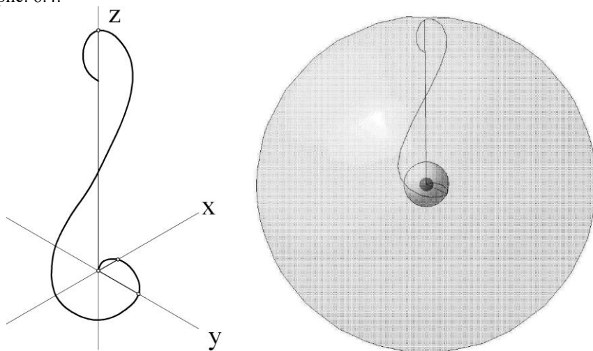
Рис. 6.4 – Принцип образования декартовой системы координат с разновеликими осями (вид слева) и с фигурой в виде скрипичного ключа, связывающей три сферы, выполненных в масштабе (вид справа)
