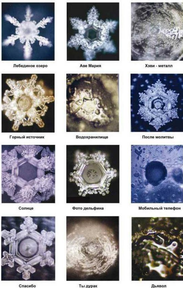
Рис. 9.5 - Изменение структуры воды под влиянием произнесенных над ней слов
