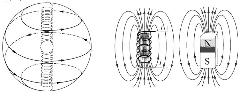
Рис. 7.2 - Силовые линии магнитного поля вихревого образования (слева), и соленоида и постоянного магнита (справа)
