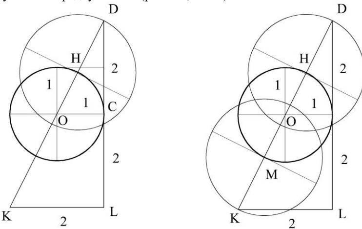
Рис. 8.3 – Стадии процесса проявления
