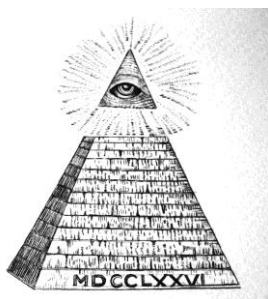
Рис. 8.19 – Пирамида с глазом наверху – древний эзотерический знак
