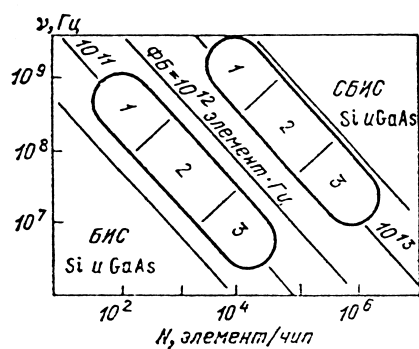
Рис. 33. Характеристики развития СВИС: 1 — ИС для управления и вычисления; 2 — радиолокационный цифровой процессор; 3 — чувствительный сигнальный процессор (Значения ФЭ области применения)
