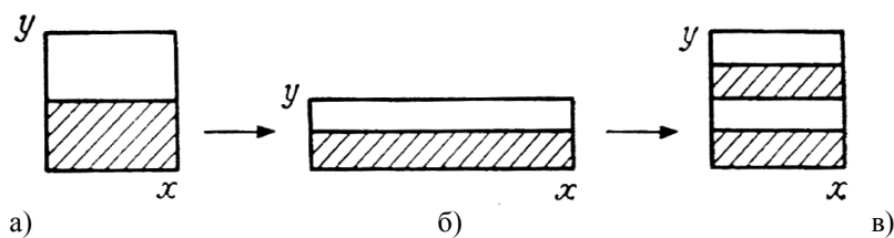
Рис. 23. Последовательные итерации преобразования пекаря приводят к фрагментированию заштрихованных и светлых полосок на все большее и большее число разъединенных областей
