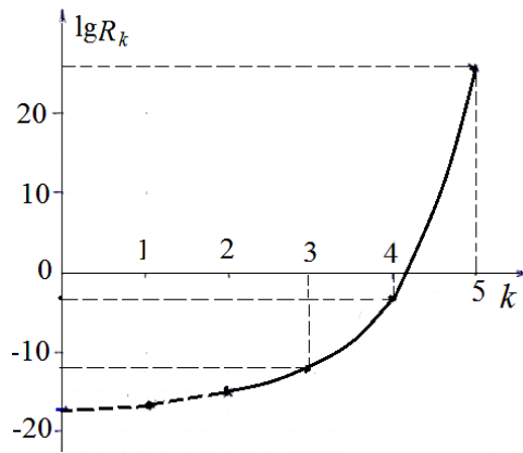
Рис. 5. График логарифмической зависимости R_k(k)
