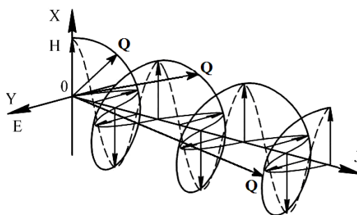
Рис. 4. Схема движения суммарного радиус-вектора Q электромагнитного импульса
