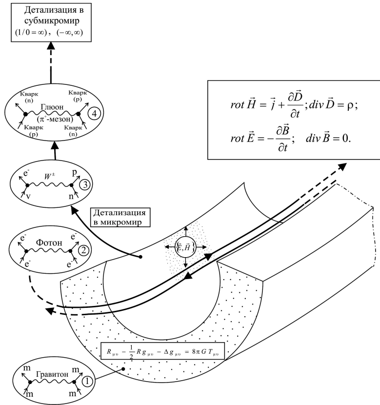
Рис. 20. Иллюстрация к вселенскому переносу информации электромагнитными волнами \{ \vec{E}, \vec{H} \} в «ложе» искривленного пространства. В уравнениях Максвелла (42): \vec{E} и \vec{D} — напряженность электрического поля и электрическая индукция; \vec{H} и \vec{B} — напряженность магнитного поля и магнитная индукция; \vec{j} и \rho — сторонний ток — источник поля и сторонний заряд, соответственно. В полевом уравнении Эйнштейна — Гильберта — Фридмана ( \Delta \neq 0 ) (43): R_{\mu\nu} — тензор Риччи (тензор кривизны Римана); R — скалярная кривизна пространства; g_{\mu\nu} — метрический тензор (функции пространственных и временных координат); \Delta — космологическая постоянная; G — гравитационная характеристика; T_{\mu\nu} — тензор энергии-импульса. Действие четырех фундаментальных взаимодействий, осуществляемых обменом квантами поля, характеризующими конкретное взаимодействие, обозначено на рисунке диаграммами Фейнмана (см., например 53 ): 1 — гравитационное взаимодействие; 2 — электромагнитное взаимодействие; 3 — электрослабое взаимодействие ( W^\pm — промежуточные частицы, W — бозоны); 4 — сильное взаимодействие (гравитон имеет спин 2, остальные переносчики взаимодействия — фотон, W^\pm и глюон — обладают спином 1)
