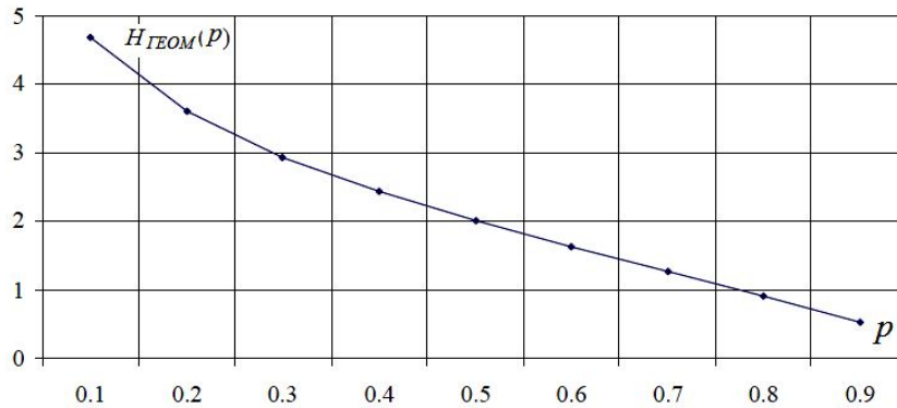
Рис. 12. Зависимость H_G(p) от параметра p
