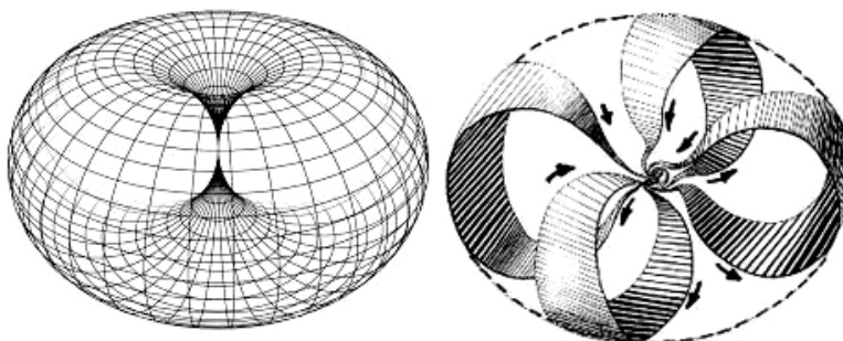
Рис. 7. Геометрия «Кляйн-тора»
