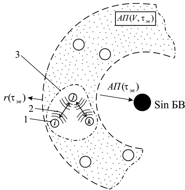
Рис. 3. Иллюстрация к теореме 2: 1 — «разумная» планета в системах «звезд главной последовательности»; 2 — взаимная ( i \leftrightarrow j ) — коммутация «разумных» планет посредством БФВ на ЭМВ; 3 — условно выделенный (для иллюстративной наглядности) ареал соседних «разумных» планет; Sin БВ — местоположение сингулярности Большого взрыва (БВ), условного центра Вселенной; AP(V, \tau_{эв}) , r(\tau_{эв}) , AP(\tau_{эв}) — см. пояснения к рис. 2, а.
