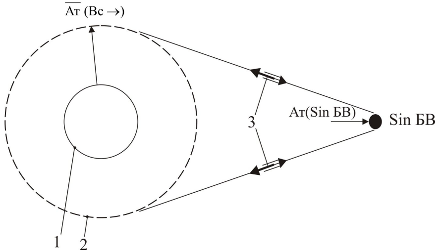
Рис. 8. Иллюстрация к гипотезе пульсирующей Вселенной: 1 — объем современной нам Вселенной; 2 — объем предельного расширения Вселенной; 3 — ходы сжатия и расширения
