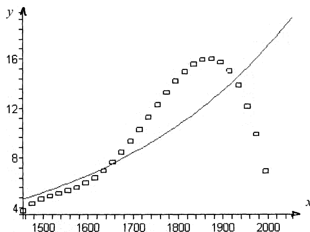
Рис. 28. Приближение аппроксимированной функции Y(x) экспоненциальной функцией
