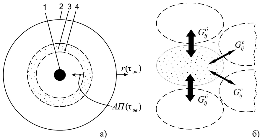
Рис. 2. К иллюстрации концепции ВВЖ: 1 — центр Вселенной — след исходной сингулярности для Большого взрыва; 2 — внешняя граница Вселенной; 3 — витагенный \equiv антропогенный пояс (АП); 4 — i -я «звезда главной последовательности» в АП (а); к возможному сценарию взаимодействий соседних вселенных в концепции их бесконечного числа (б)
