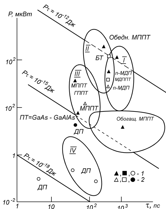
Рис. 32. Диаграмма: рассеиваемая мощность — время переключения ( P - \tau ) для АЭ различных типов: 1 — характерные точки для АЭ: полевых транзисторов (ПТ), биполярных транзисторов (БТ), джозефсоновских переходов (ДП); 2 — расчетные точки для тех же АЭ (МДП — металл-диэлектрик-проводник, МП — металл-полупроводник, ГП — гетеропереход). На рисунке изображены области параметров, характерных для ПТ со структурой металл-диэлектрик-полупроводник (МДППТ) — I, со структурой металл-полупроводник (МППТ) — III, для БТ — II, для ДП — IV
