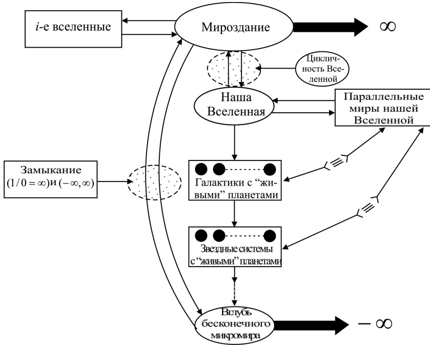
Рис. 15. Иллюстрация к теореме 4: общая структура «живого» Мироздания с замыканием в себе (1/0 = \infty) и (-\infty, \infty) ; \Leftrightarrow означает равнозначие, то есть идентичность «нашего» и параллельных миров
