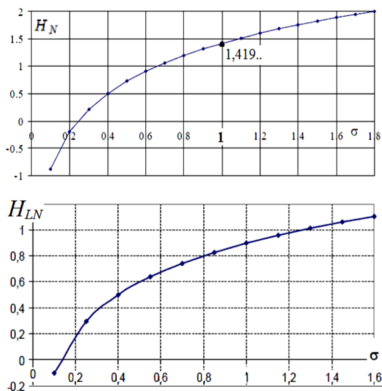
Рис. 14. Зависимость дифференциальной энтропии H_N нормального и H_{LN} логнормального распределения от параметра \sigma , превратившегося в параметр формы H_{LN}
