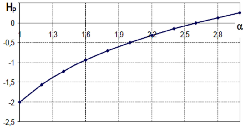
Рис. 13. Зависимость дифференциальной энтропии распределения Парето от параметра \alpha при b=1
