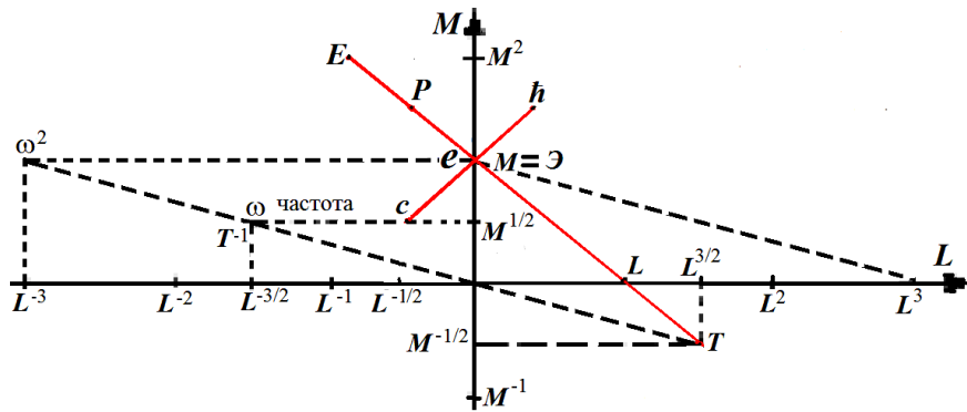
Рис. 6. Соотнесение массы и длины
