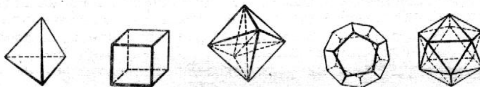
Рис.6. Пять правильных многоугольников. Слева направо: Тетраэдр. Гексаэдр или куб. Октаэдр. Додекаэдр. Икосаэдр
