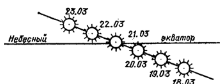
Рис. 4. Переход Солнца через точку весеннего равноденствия \gamma [4, с. 14].
