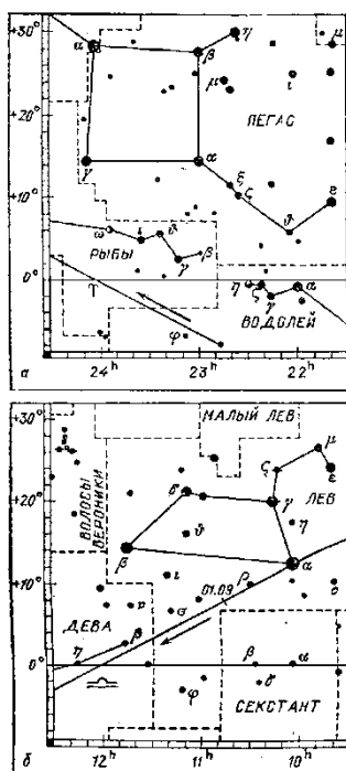
Рис. 3. Положение точки весеннего равноденствия \gamma (а) и точки осеннего равноденствия \omega (б) на небесной сфере. По горизонтали отложено прямое восхождение \alpha , по вертикали – склонение \delta ; стрелкой указано направление движения Солнца по эклиптике; дата 01.09 на рис. б указывает положение Солнца на начало сентября [4, с. 13].
