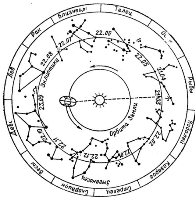
Рис. 24. Круг зодиакальных созвездий [4, с. 40].
