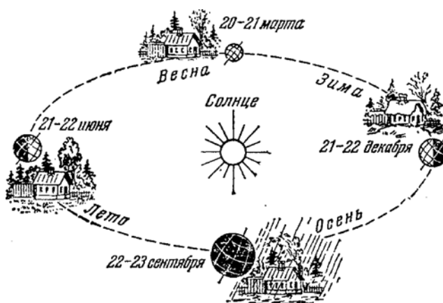
Рис. 22. Движение Земли вокруг Солнца и смена времен года [4, с. 37].
