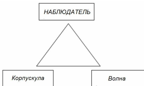
Рис. 2. Ситуация квантового парадокса "Наблюдатель"
