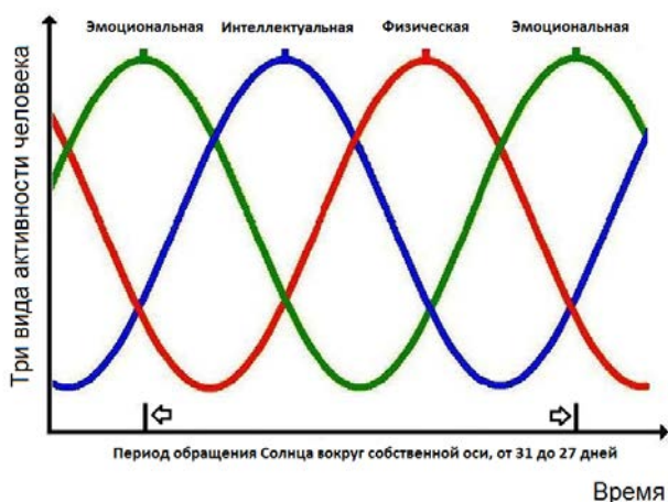
Рис.30 а). Колебание склонностей сбалансированной, гармоничной личности, — «ритмика» (см. рис.31 а)). Триадный цикл активности человека связан с обращением Солнца вокруг своей оси. Период цикла меняется от максимального значения (31 день) в начале 11-летнего цикла солнечной активности до минимального значения (27 дней) в конце 11-летнего цикла.
