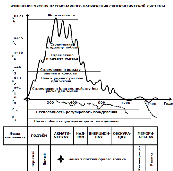
Рис.25. Изменение пассионарного напряжения этнической системы (обобщение).
