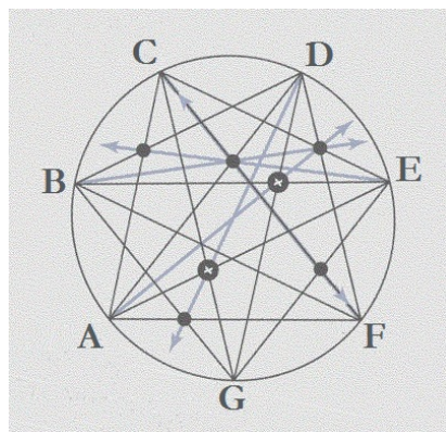
Рис.10. Вариант совершенного сада камней. Из точки G видны все семь камней. Крестиками обозначены два камня, которые всегда видны в любой из семи позиции для созерцания A – G.
