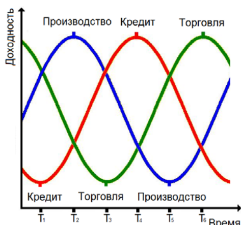
Рис.21 а). Триадное взаимодействие отраслей экономики.
