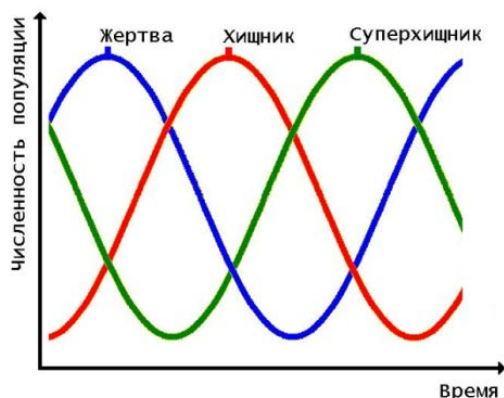
Рис.19. Вариант решения СДУ Жертва-Хищник-Суперхищник – периодические колебания.
