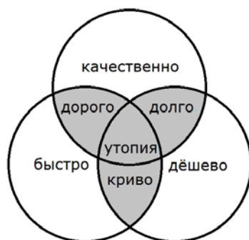
Рис.6. Диаграмма Венна, иллюстрирующая закономерности «магического треугольника».
