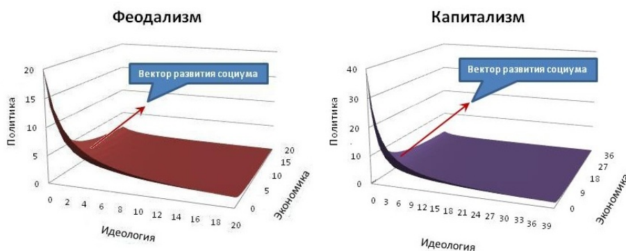
Рис.12. Плоскости состояний социума, являющиеся решениями уравнения Политика * Идеология * Экономика = E . Чем сложнее социум, тем больший объём энергии «E» он контролирует.
