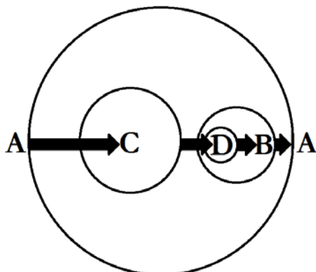
Рис.11. Схема описанного в произведении С. Норки циклического нетранзитивного контроля: A \rightarrow C \rightarrow D \rightarrow B \rightarrow A .
