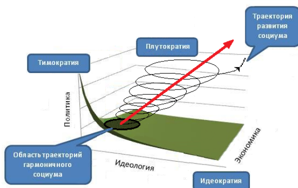
Рис.13. Схематическое изображение области существования, воронки развития и предельных состояний социума.
