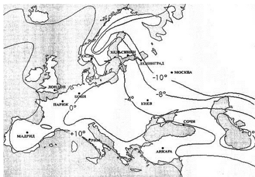
Рис.27. Изотермы (линии равных температур) января на территории Европы (построены на основании климатических карт "Атласа офицера" (М.Воениздат, 1978г.) и Большого настольного атласа Маркса (М., зд-во Маркса, 1904 г.).
