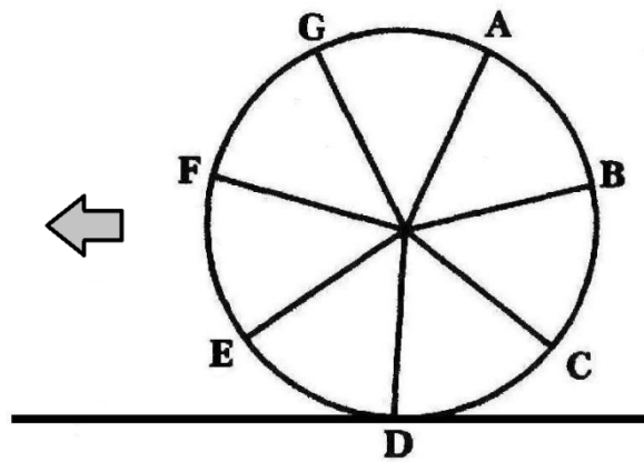
Рис.22. Качение колеса – пример циклического перехода причины в следствие и обратно.
