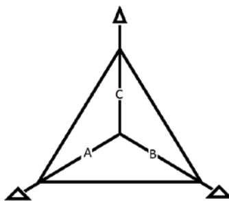
Рис.4. Пирамида, построенная на трёх ортах как на рёбрах.
