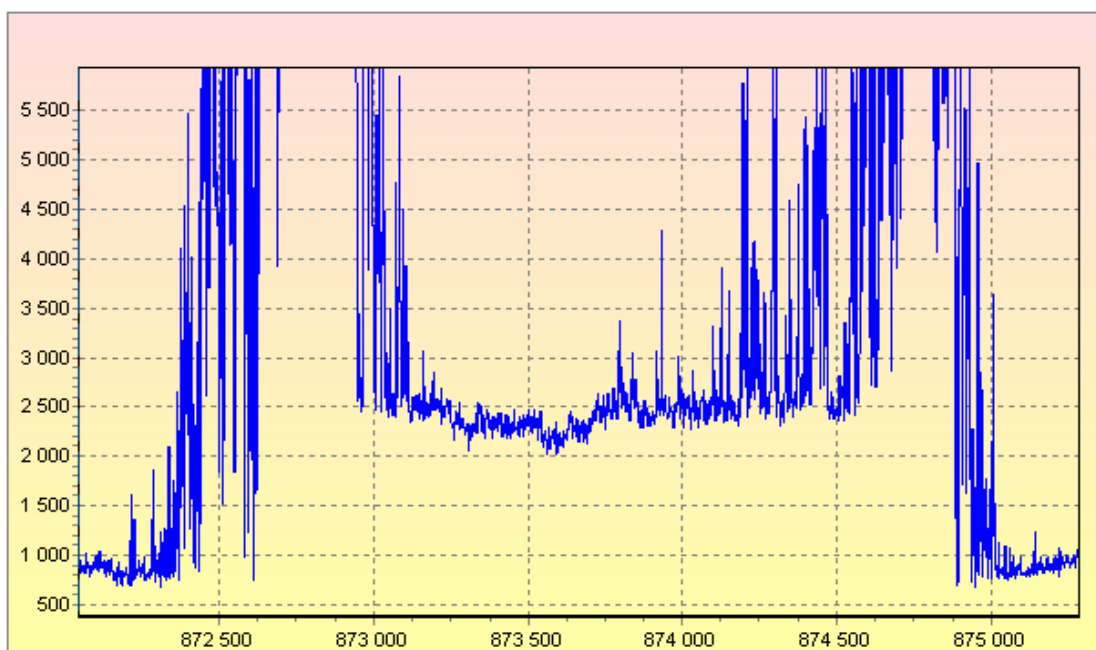
Рис. 28. Торсионный предвестник землетрясения на Суматре.
