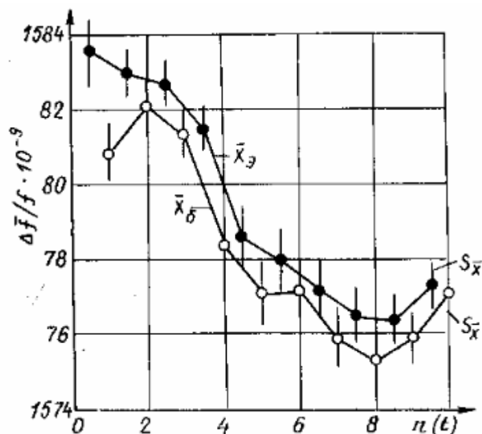
Рис. 19. Воздействие спирного поля на кварцевый резонатор через 8-слойный алюминиевый экран: n(t) – количество циклов усреднения (1 цикл – 200 с). X_3 – среднее арифметическое при воздействии через экран; X_6 – среднее арифметическое при воздействии без экрана; S_x – ошибка среднего (Рис. 3 из [53]).
