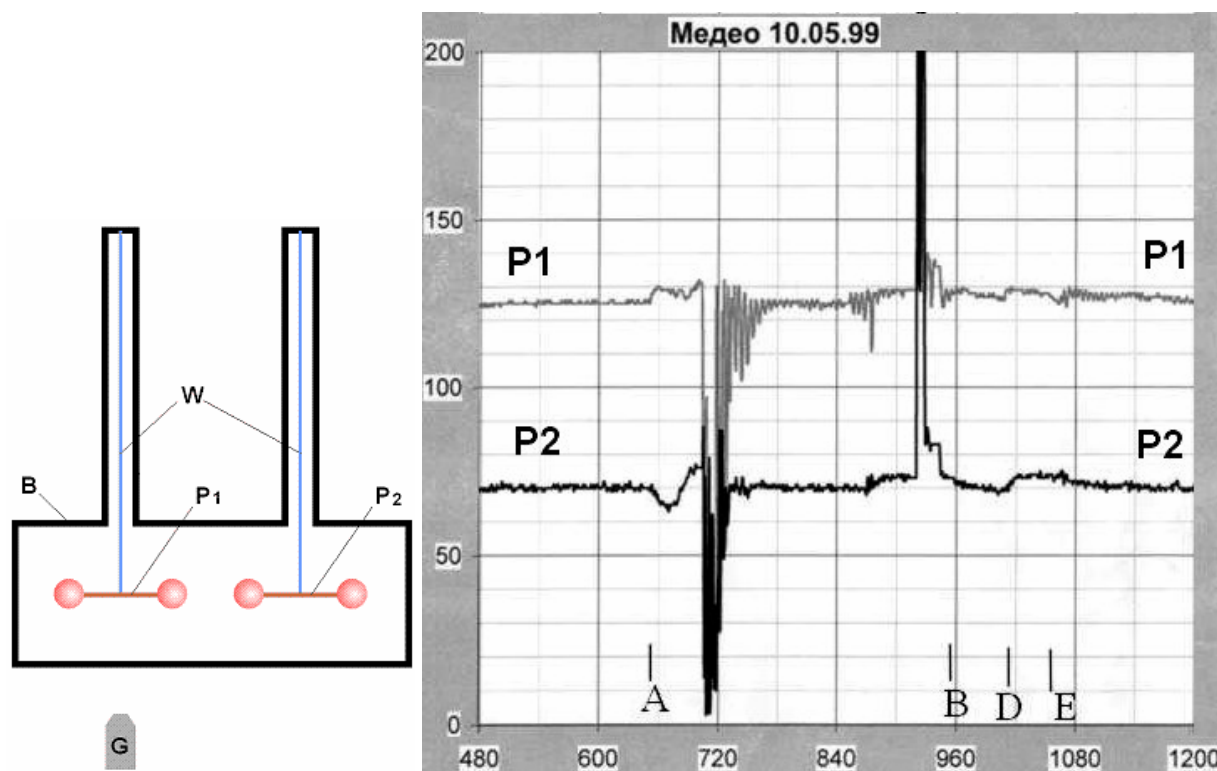
Рис. 10. Схема эксперимента А.А.Шпильмана с маятником кручения и зарегистрированные отклонения маятников http://www.spinfields.hut2.ru/ALMANACH/2n01/Medeo.htm .
